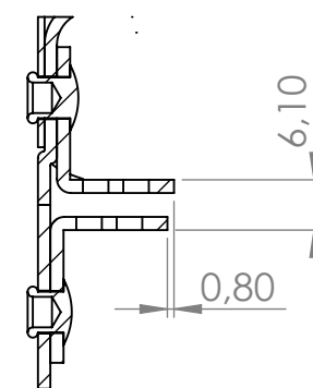
SCHNITT A-A MAßSTAB 1 : 1
